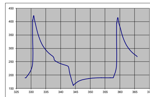
Temperatura jako funkcja czasu na powierzchni matrycy
