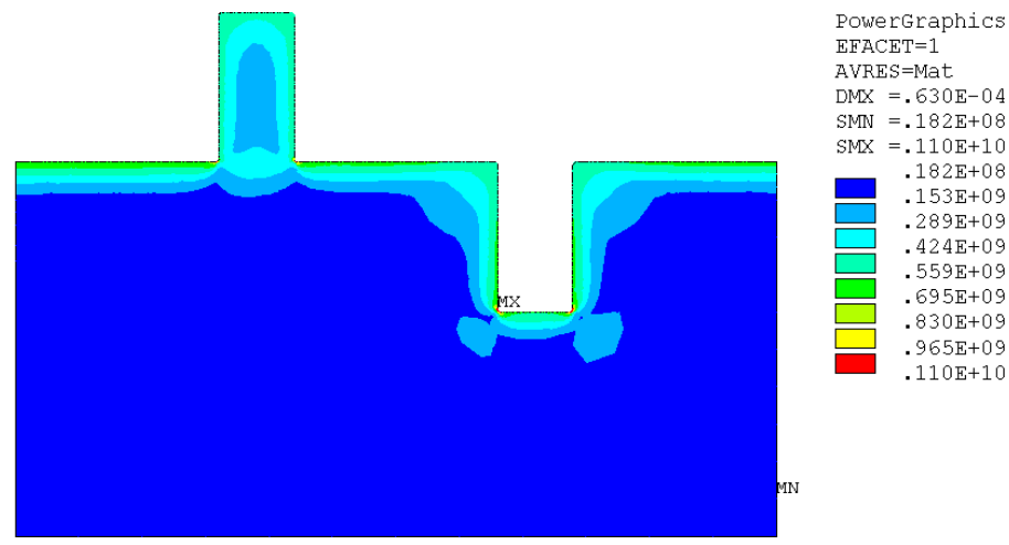
Rozkład naprężeń von Misesa w czasie tx. Promień karbu R=0,5 mm
