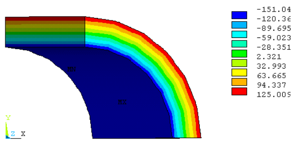
Rozkład naprężeń na ścieżce AB
